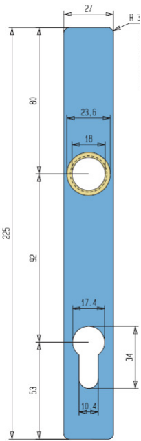
2) Langschild aussen - Profilzylinder
